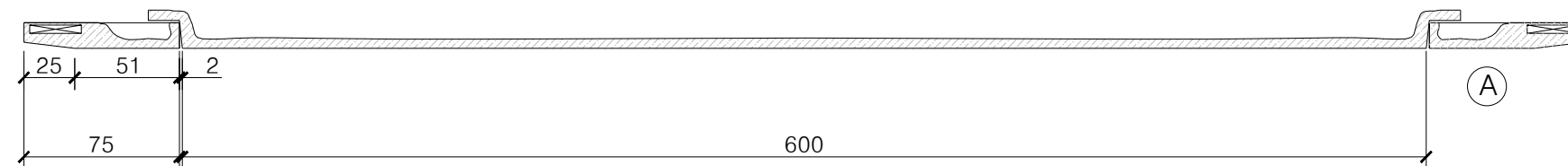
SECTION A-A
